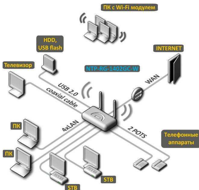
Рисунок 1 – Схема применения NTP-RG-1402
