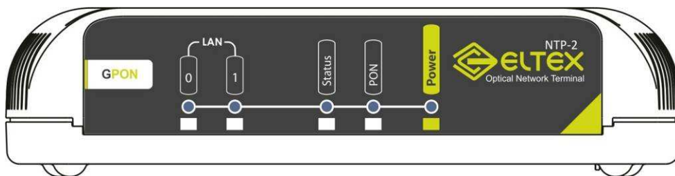
Рисунок 2 – Передняя панель абонентского терминала NTP-2
